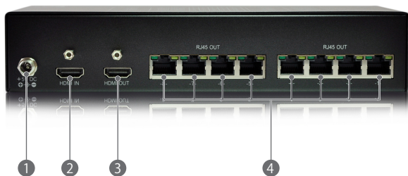
ET-HST8300 送信機：背面図
