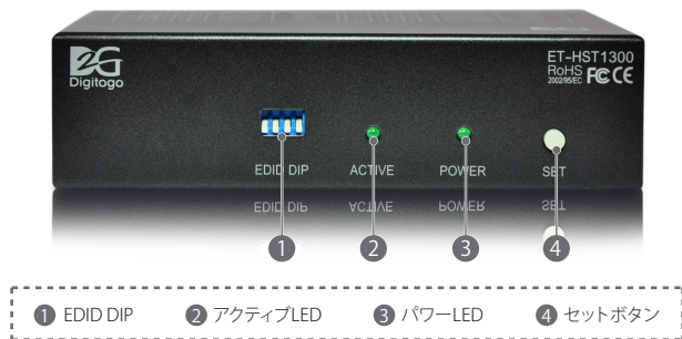
ET-HST1300 送信機：前面図
