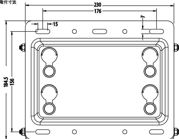
壁面取付寸法
