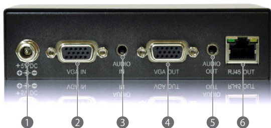
ET-VST1300 送信機:背面図
